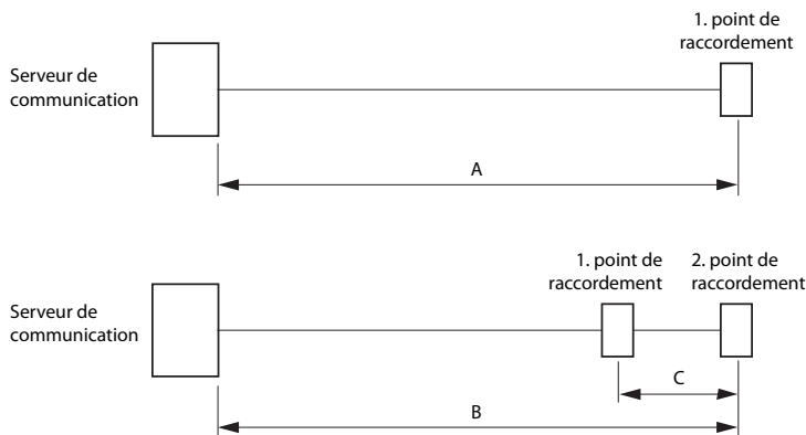
Fig. 46 Bus DSI-AD2
