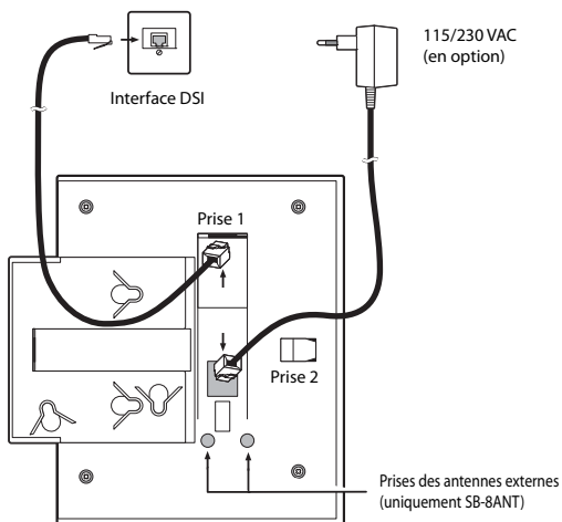
Fig. 72 Dos des unités radio avec points de raccordement
