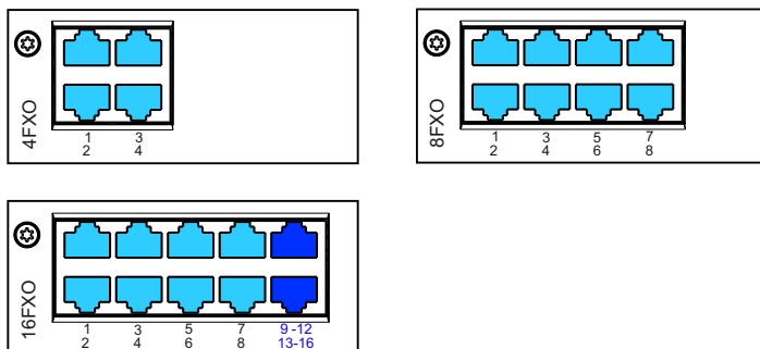
Fig. 44 Possibilités de raccordement des interfaces réseau FXO
